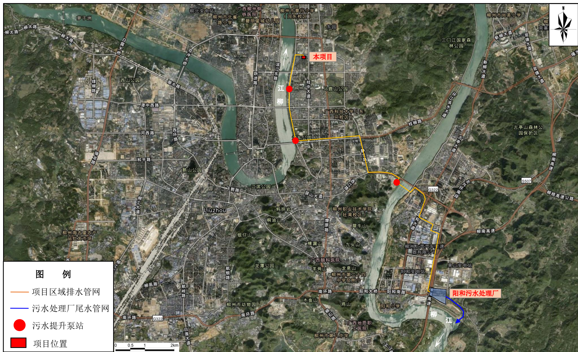
附图 8 项目区域排水管网示意图
