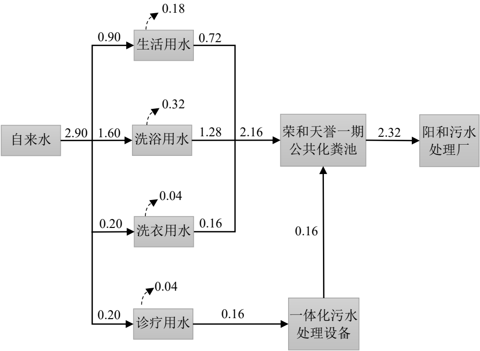
图 2-1 项目用水平衡图 单位：m³/d
